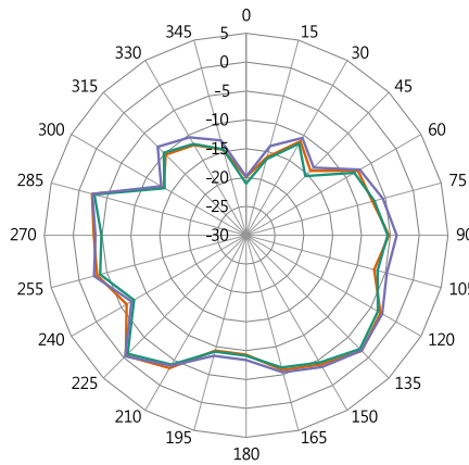
YZ-Plane Gain
