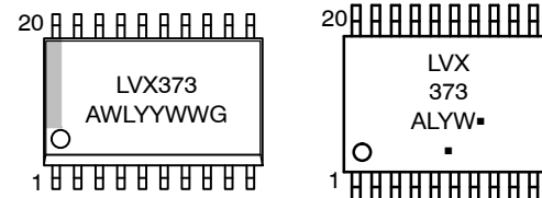
SOIC-20
